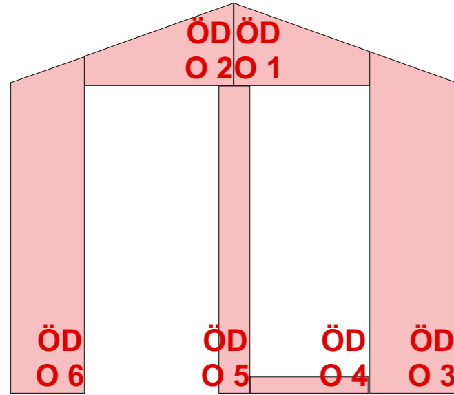
Bina İçinden Ön Duvar Paneli İç OSB Kaplamalar
