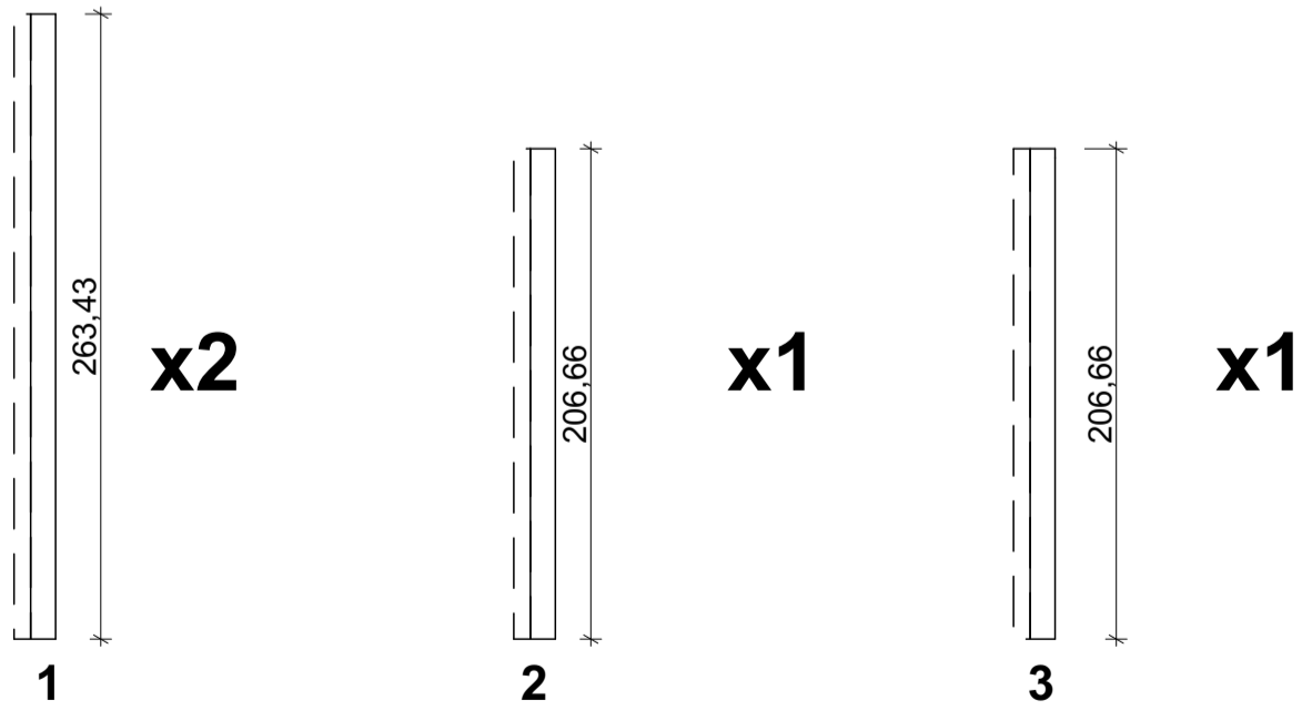
Sac L Profil Kaplama (Arka Cephe) 10cm x 10cm
